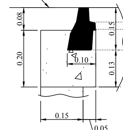
ΛΕΠΤΟΜΕΡΕΙΑ "Β"
