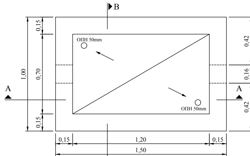
ΚΑΤΟΨΗ
