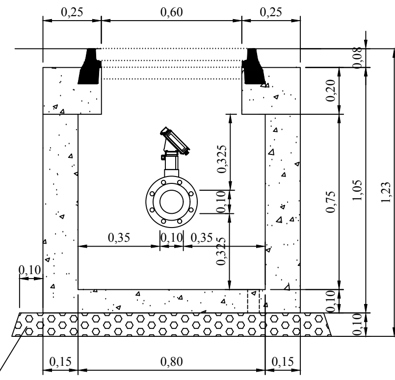
ΤΟΜΗ Β-Β
