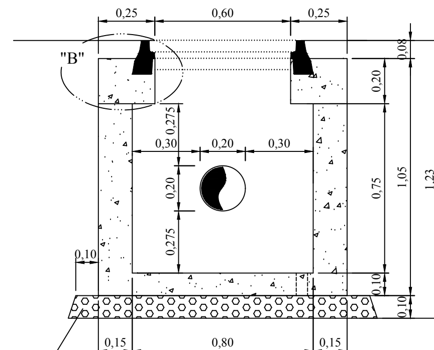
ΤΟΜΗ Β-Β
