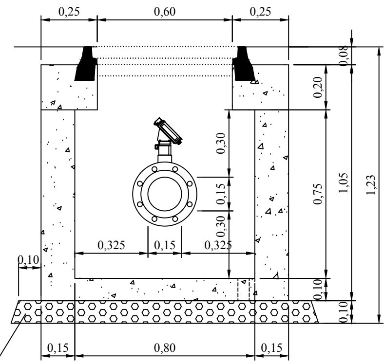
ΤΟΜΗ Β-Β
