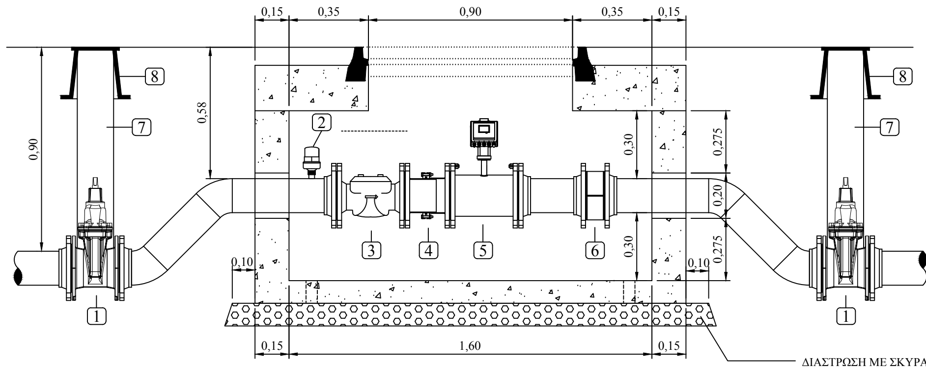
ΤΟΜΗ Α-Α
