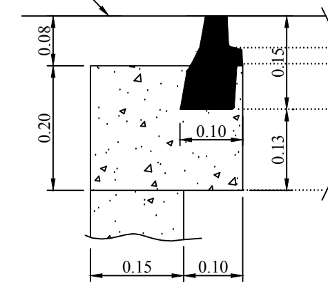
ΛΕΠΤΟΜΕΡΕΙΑ "Β"
