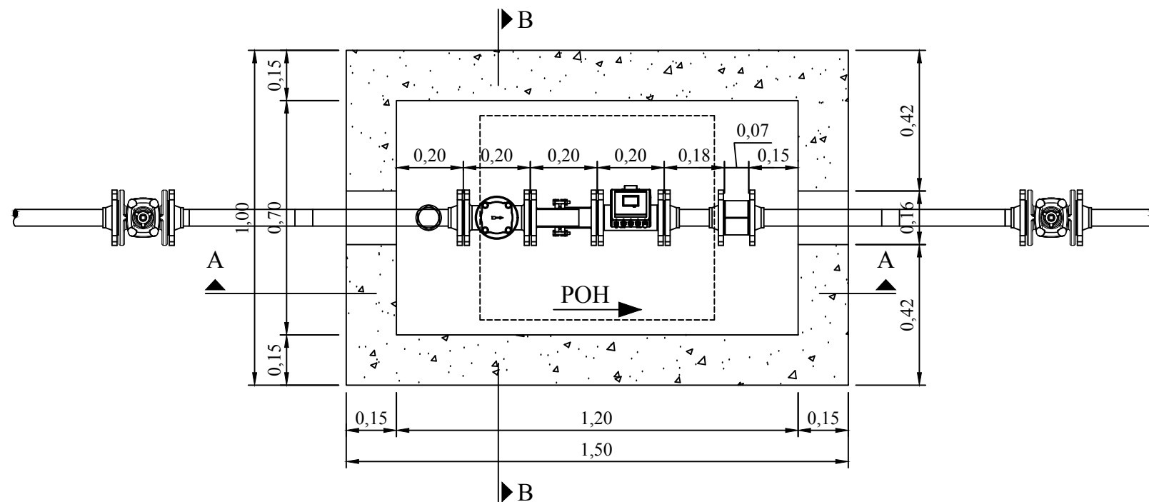
ΚΑΤΟΨΗ
