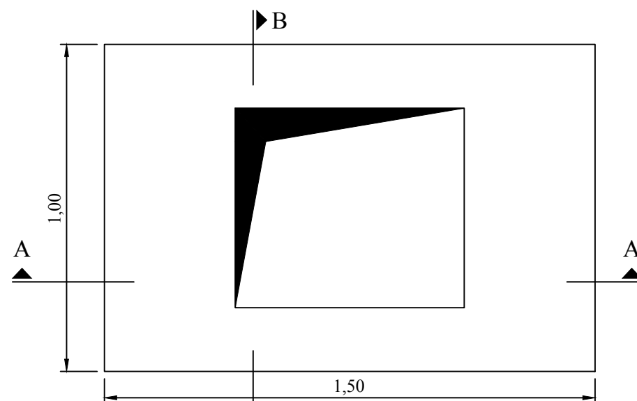
ΠΛΑΚΑ ΟΡΟΦΗΣ
