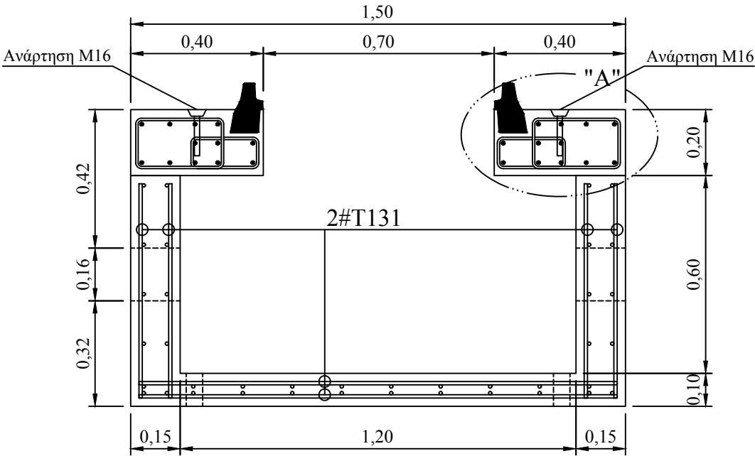
ΤΟΜΗ Α-Α
