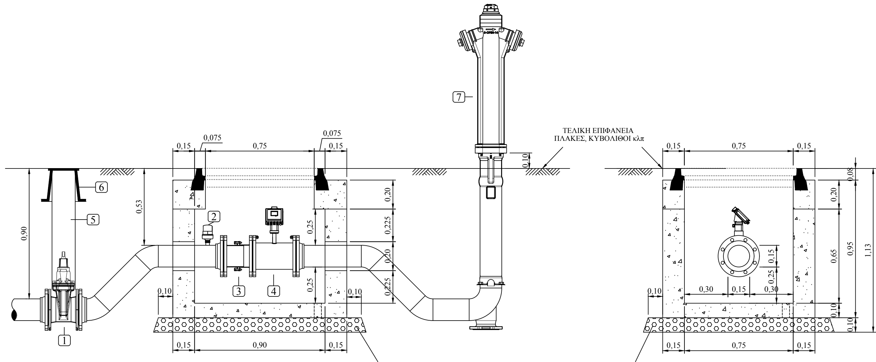
ΤΟΜΗ Β-Β
