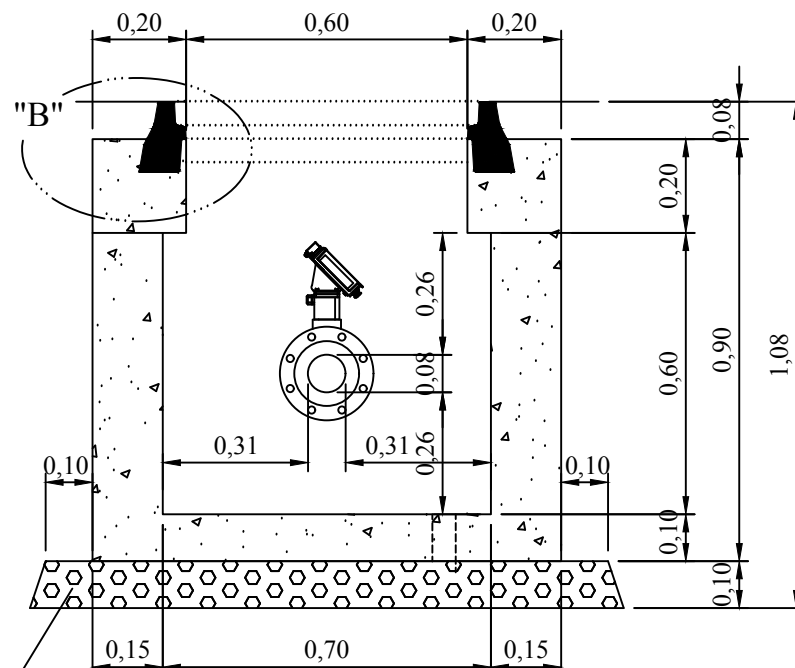
ΤΟΜΗ Β-Β
