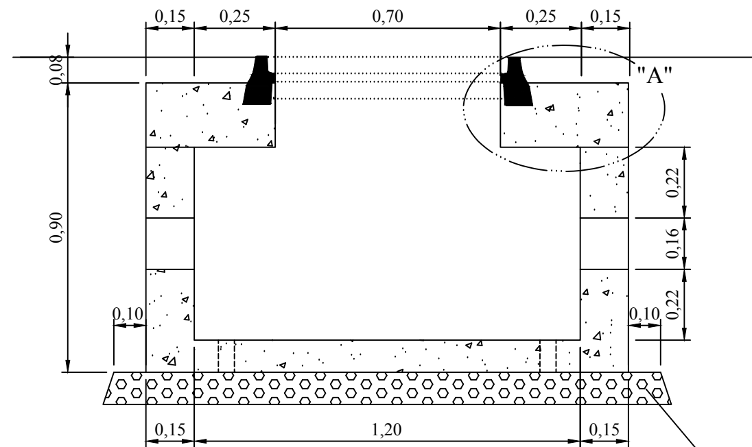
ΤΟΜΗ Α-Α
