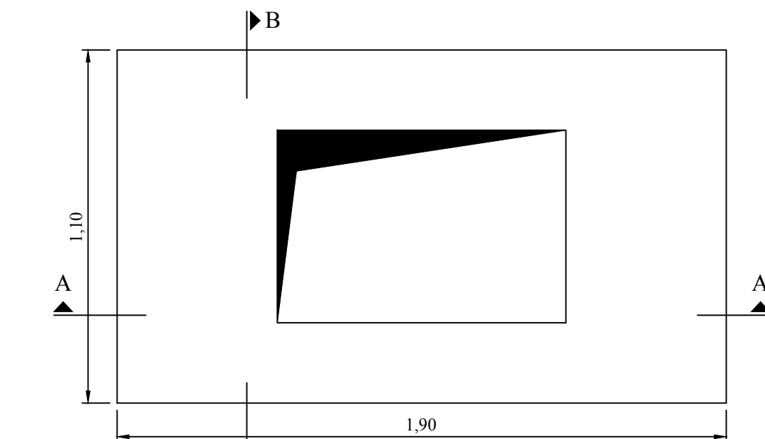
ΠΛΑΚΑ ΟΡΟΦΗΣ
