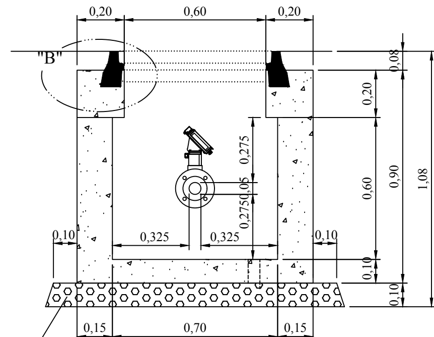
ΤΟΜΗ Β-Β
